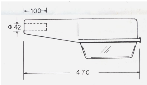
Ενδ. διαστάσεις φωτιστικών σωμάτων οδικού φωτισμού 150W
